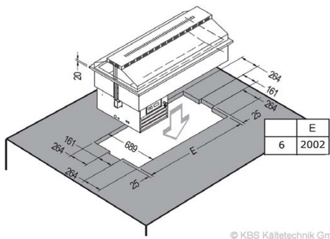
Einbauskeizze
